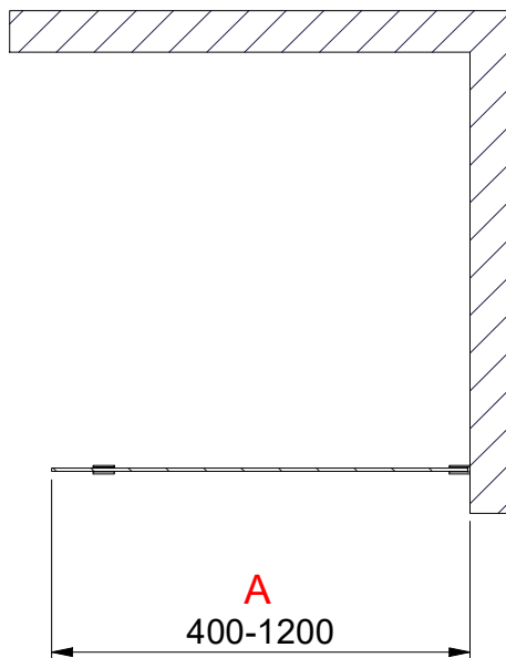
A-A ( 1 : 20 )
