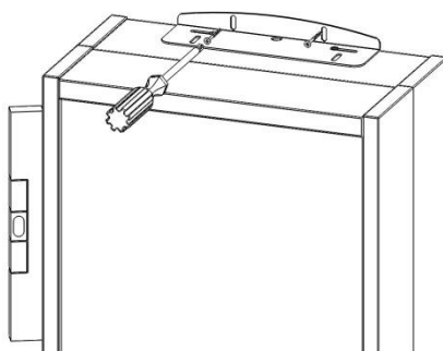
Skruva fast den övre vinkeln mot väggen
