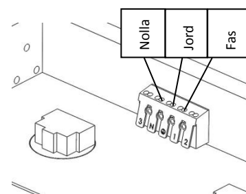
Alt. För El installation
